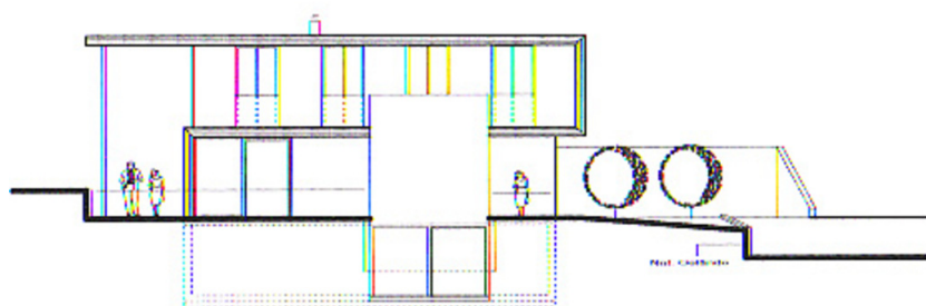
Ansicht - Süd
