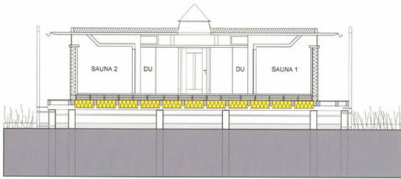
SCHNITT A-A
