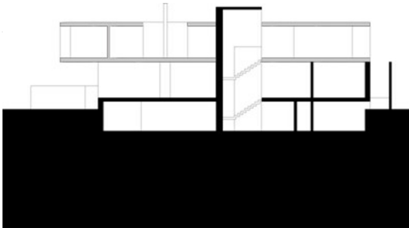
Schnitt
