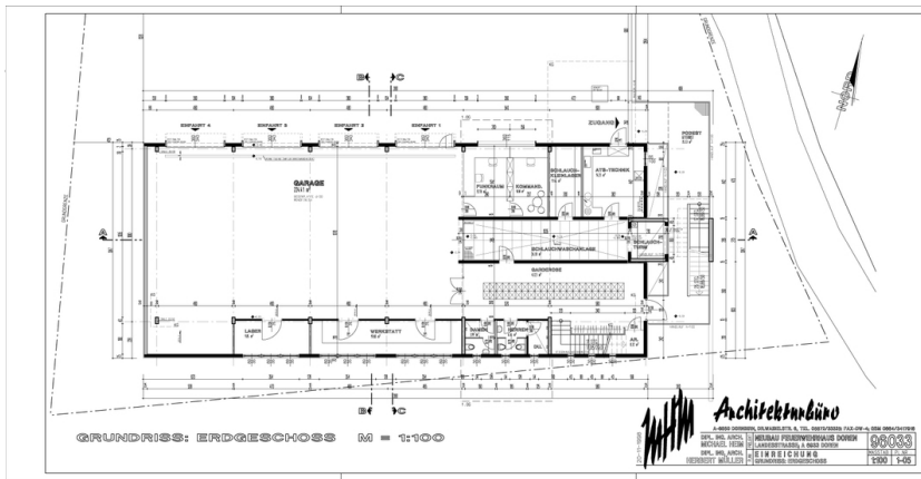
Grundriss EG
