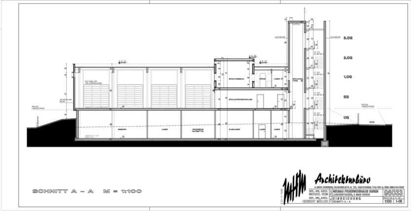
Schnitt
