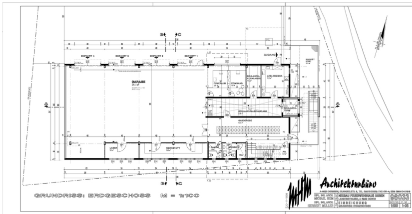
Grundriss EG
