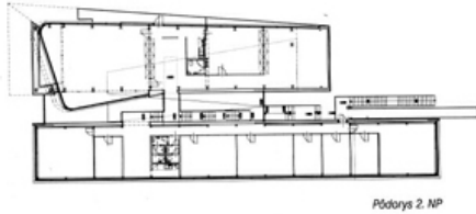
Pódorys 2. NP
