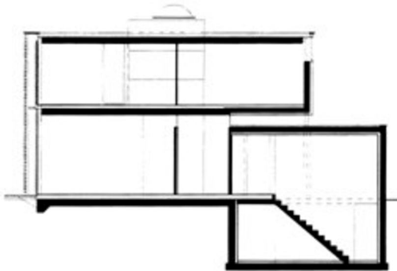
Schnitt
