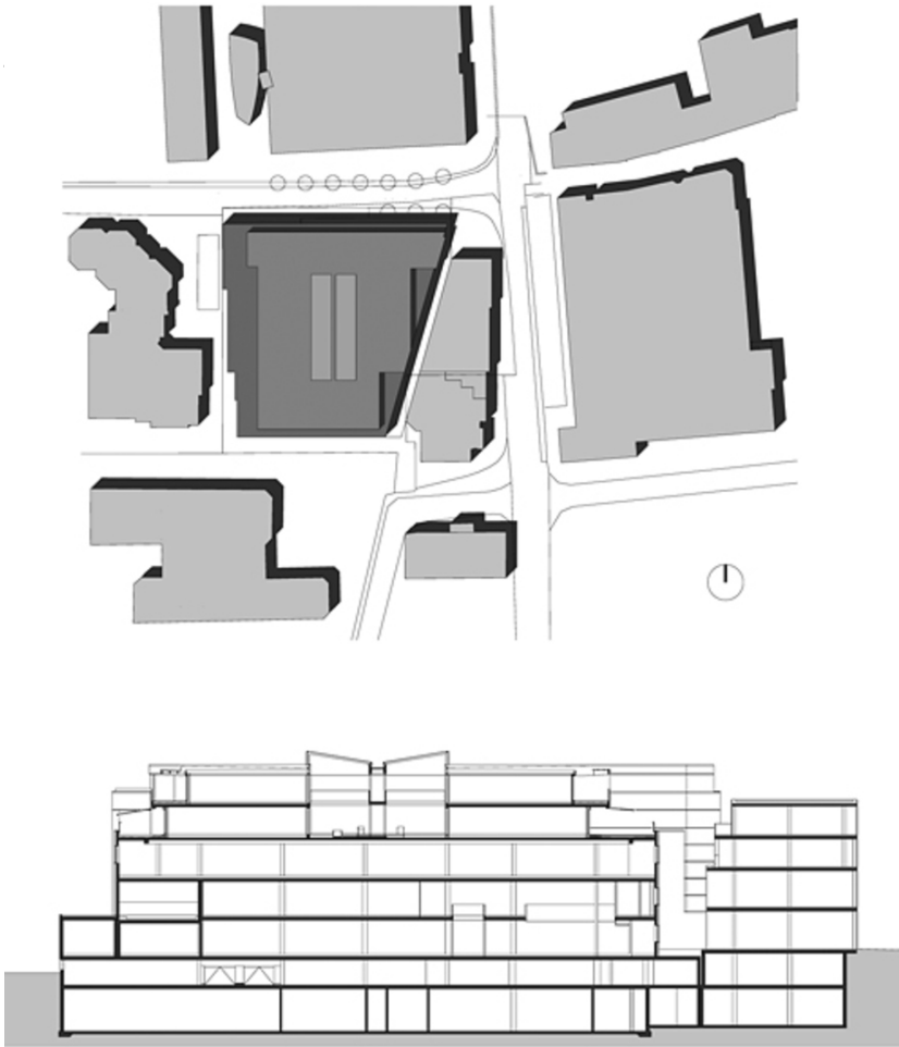
Lageplan, Schnitt
