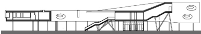
Schnitte / Ansichten
