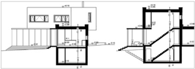
Schnitte
