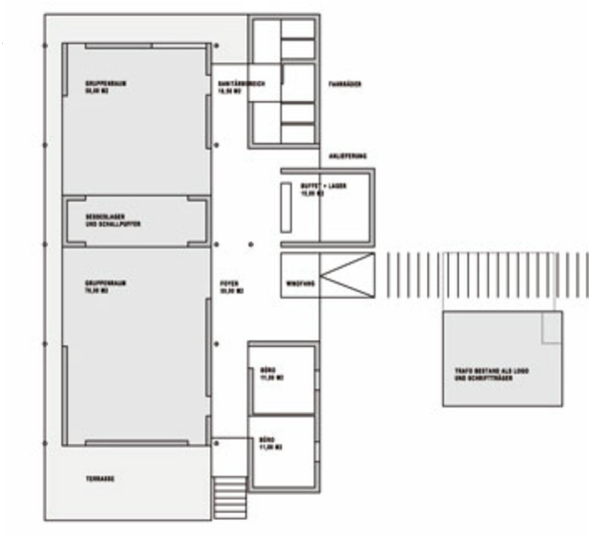
Grundriss
