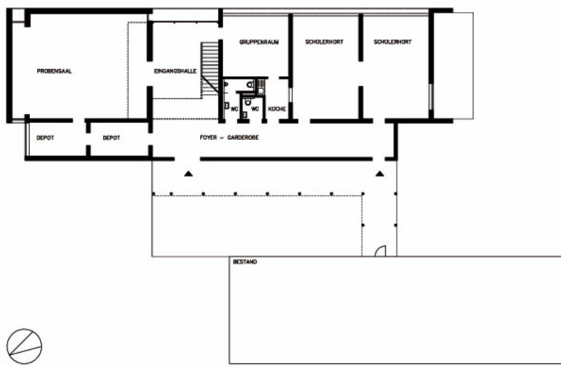
Grundriss EG
