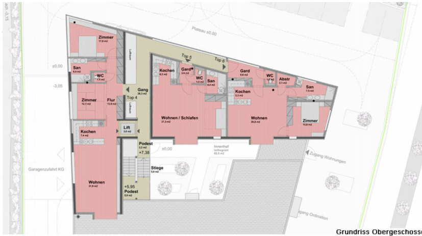
Grundriss Obergeschoße
