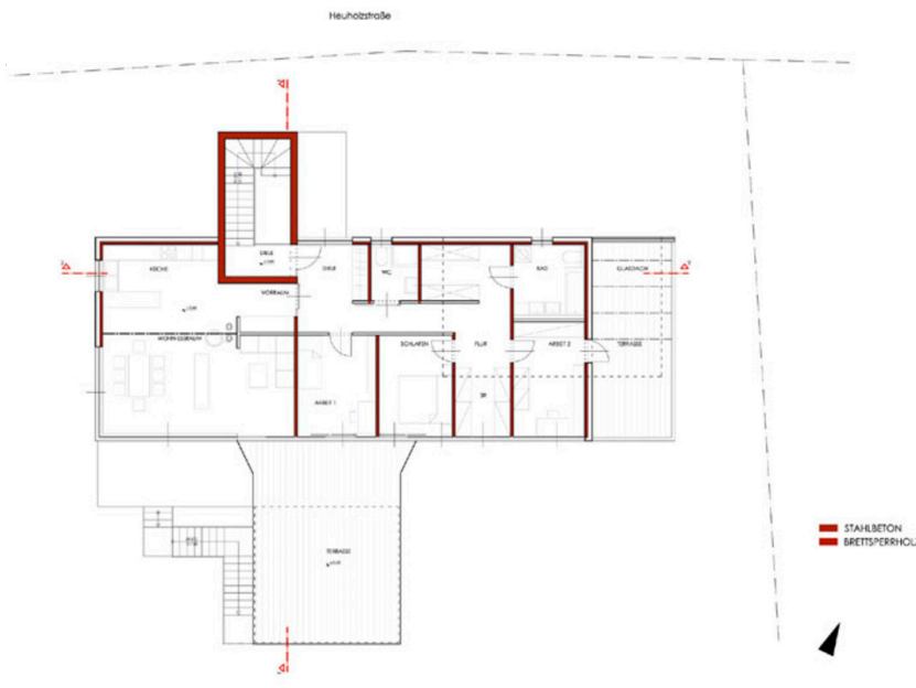
Grundriss OG
