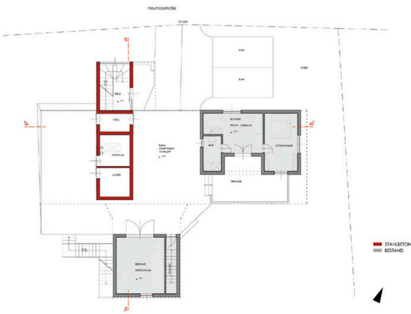
Grundriss EG
