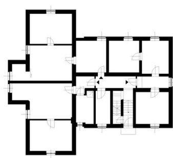
GRUNDRISS BESTAND
