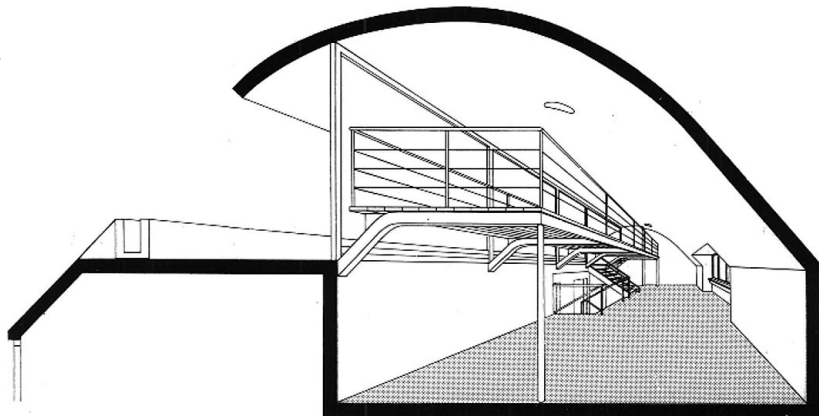
Schnitt Dachwohnung
