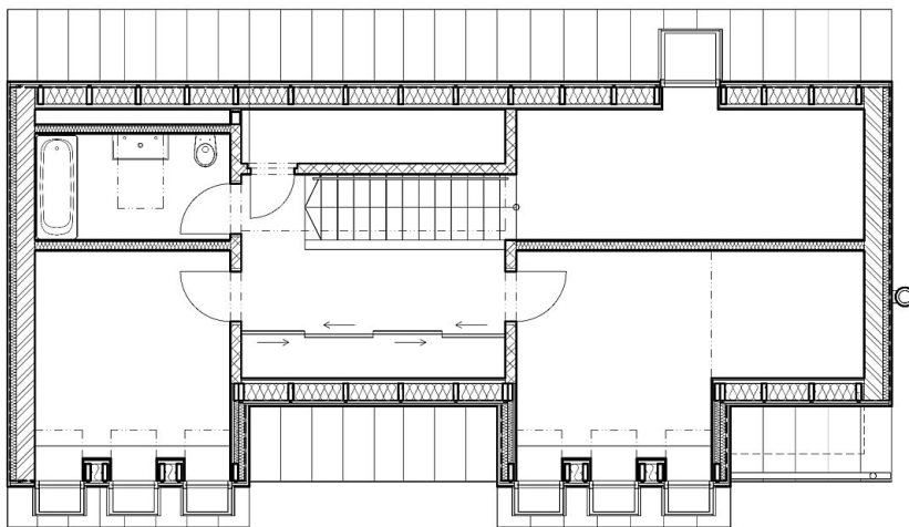
PŇDORYS PODKROVIA
