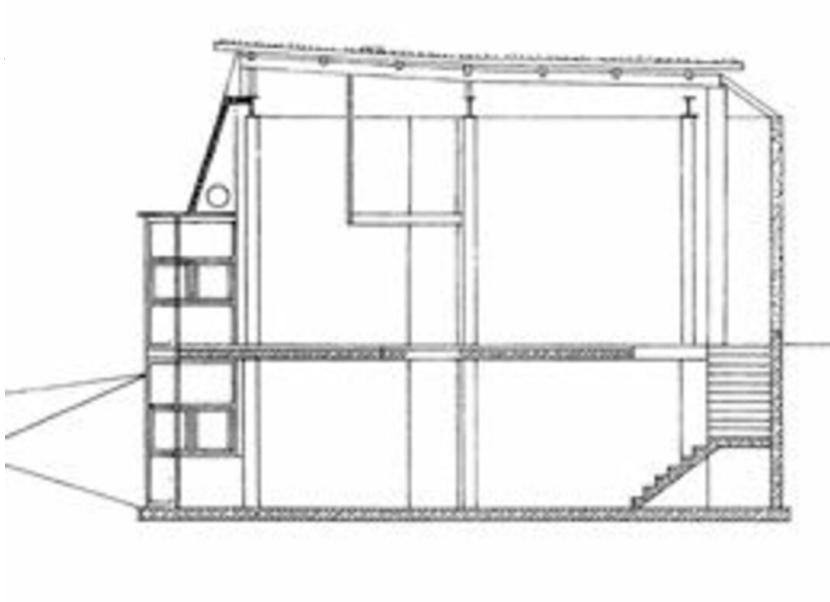
Längsschnitt
