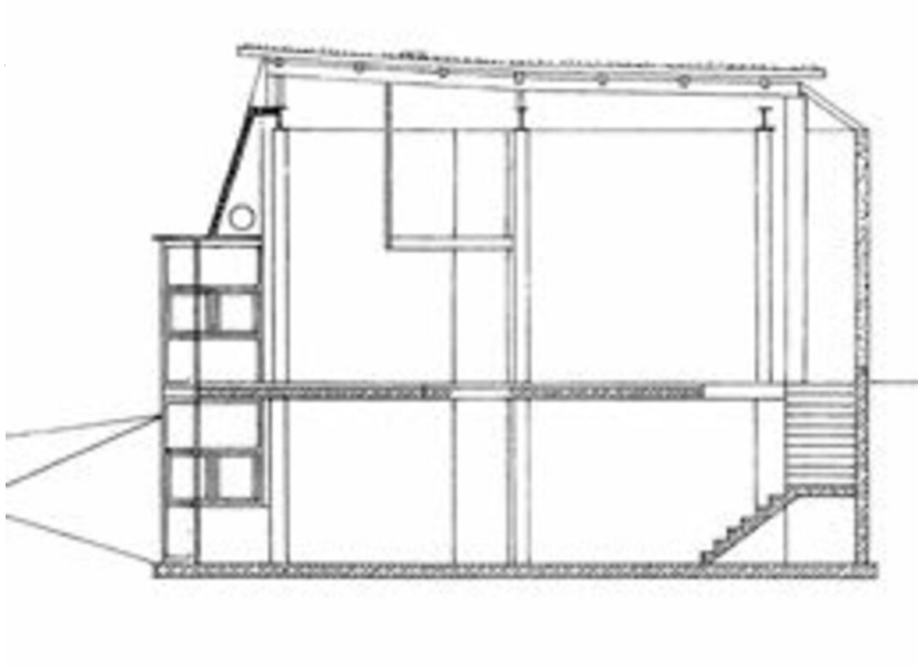
Längsschnitt
