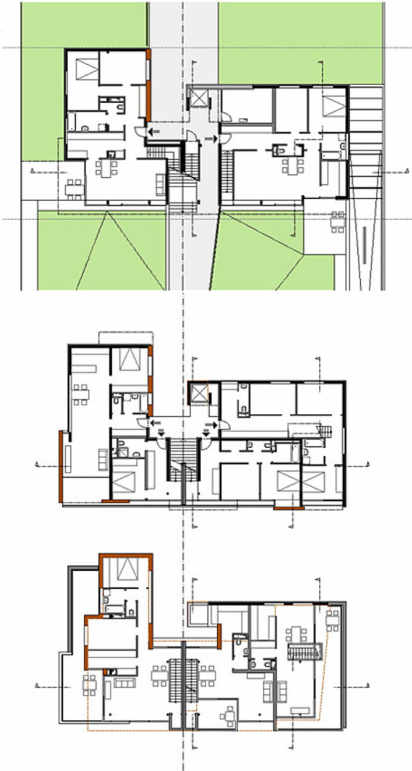
Grundriss
