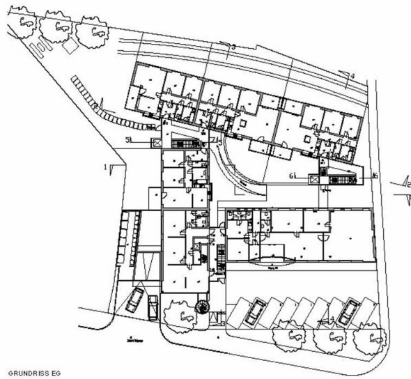
GRUNDRISS E0
