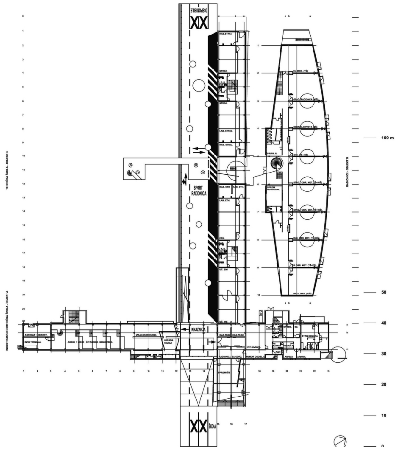
Grundriss EG
