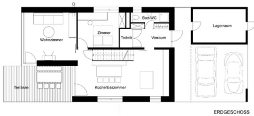
Grundriss
