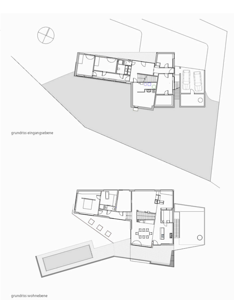
grundriss wohnenebene
