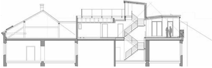
Dachausbau Neustiftgasse
