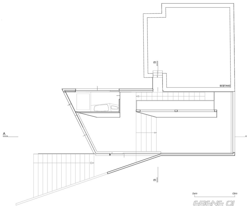
Grundriss Ebene 01
