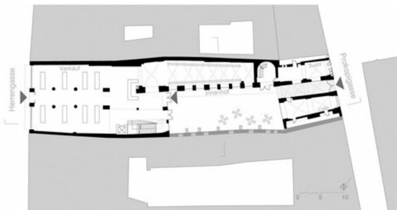
Grundriss
