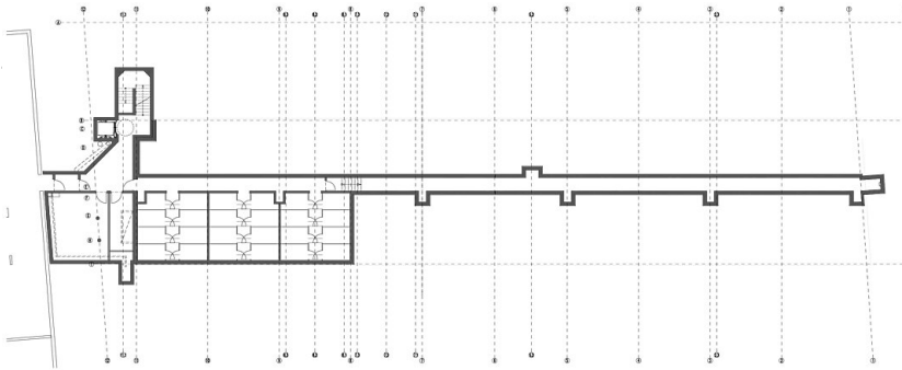
Generationen: wohnen am mühlggrund - architekten cooeh, kirschnitz, newirth - wien, 2011 / BT III, arch. cooeh - grundriss obergeschoss
