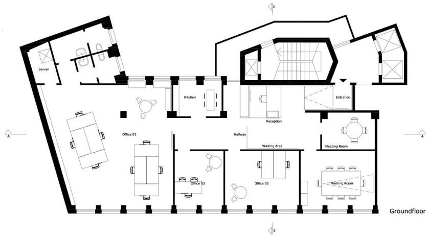
Grundriss
