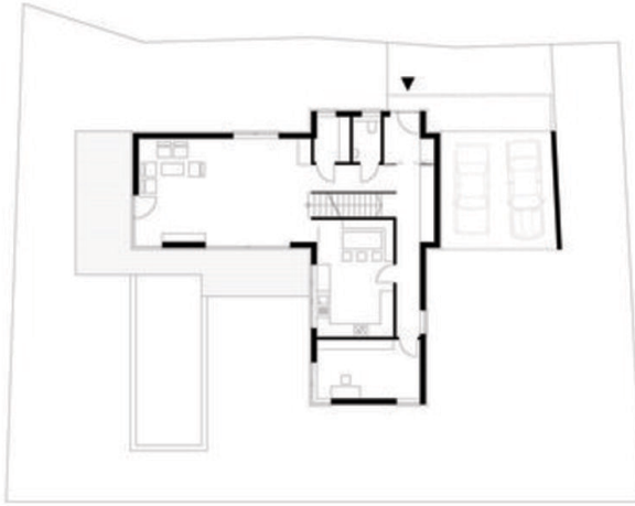
EG Haus 04
