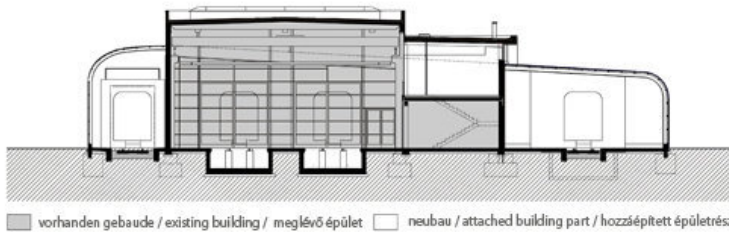
schnitt AA / section AA / AA metszet
