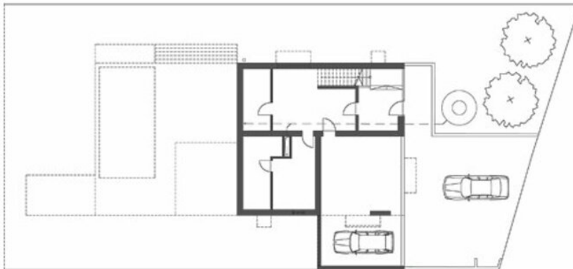
Grundriss
