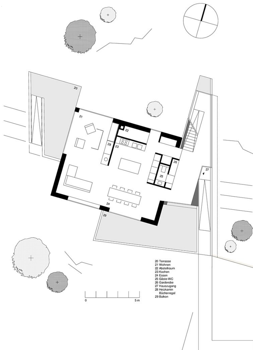
Grundriss Erdgeschoss
