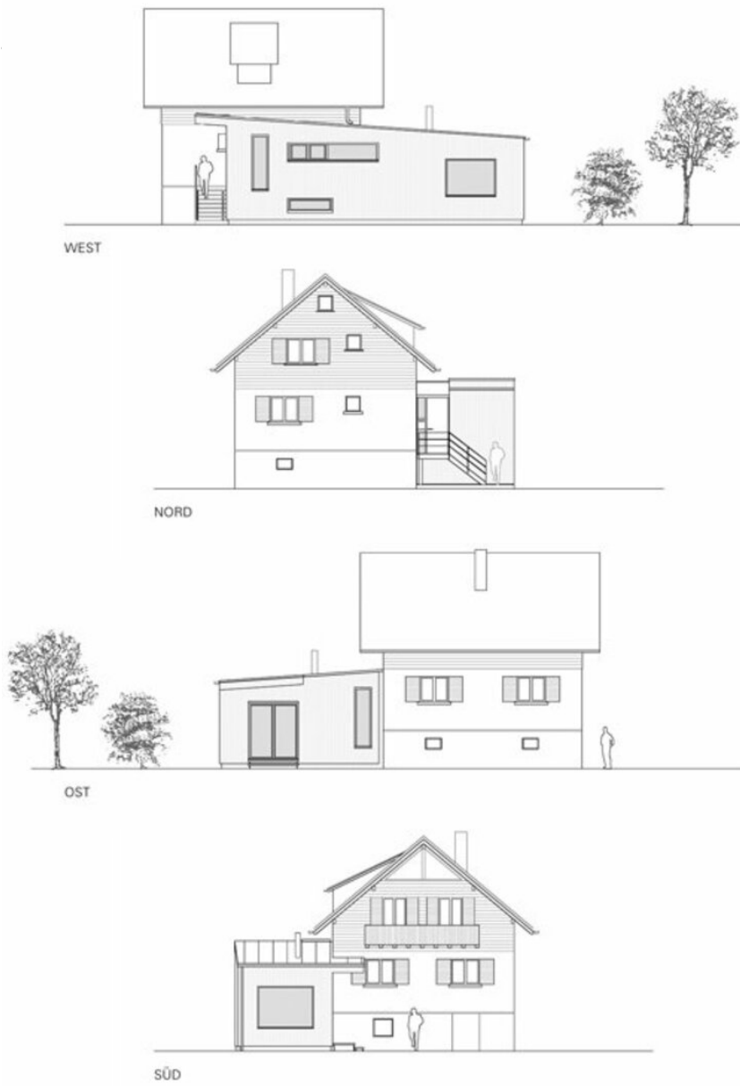
Ansichten
