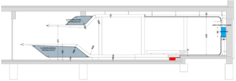
SCHNITT B-B
