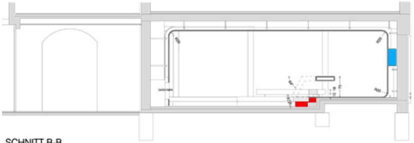
SCHNITT B-B
