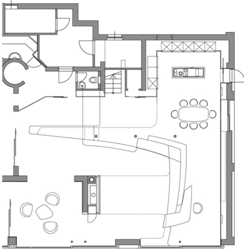
Grundriss EG
