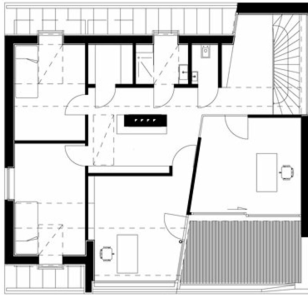
Grundriss DG
