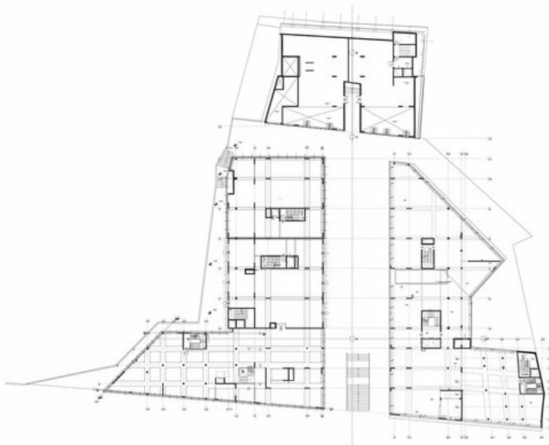
Grundriss OG1
