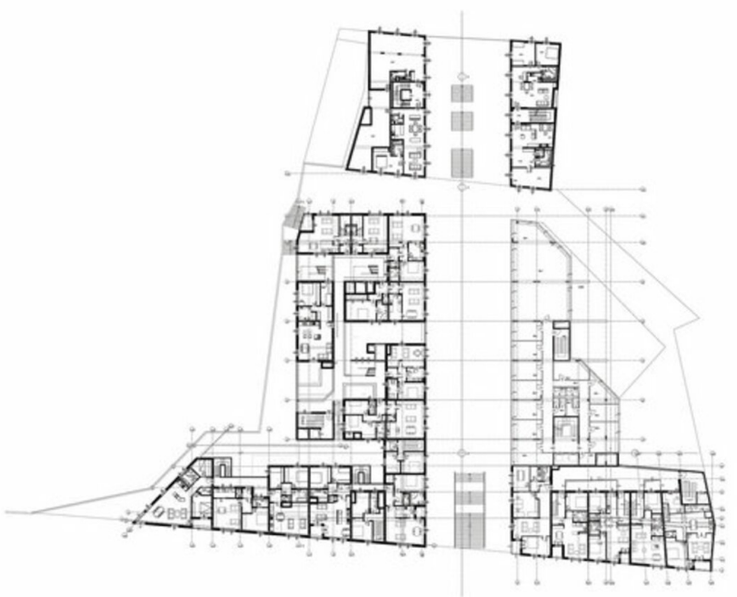
Grundriss OG4
