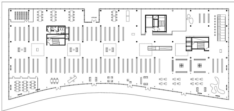
2.OBERGESCHOSS M 1:500
