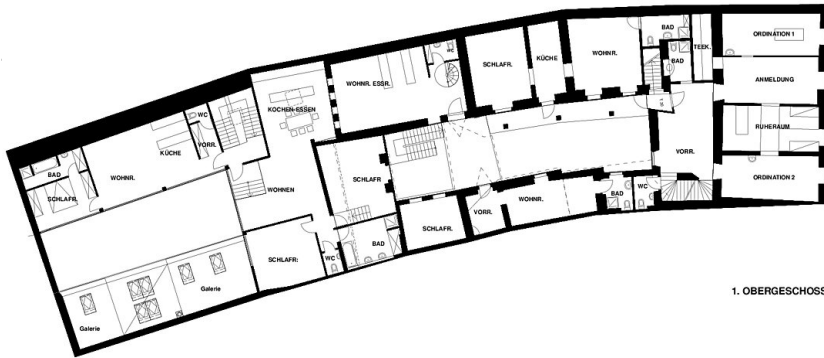
1. Obergeschoß
