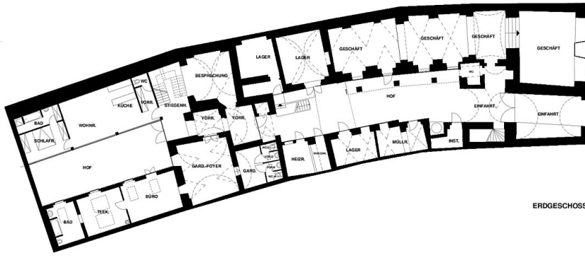
Erdgeschoß
