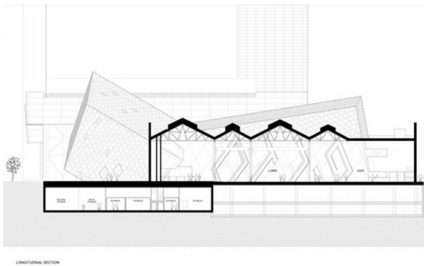
Längsschnitt
