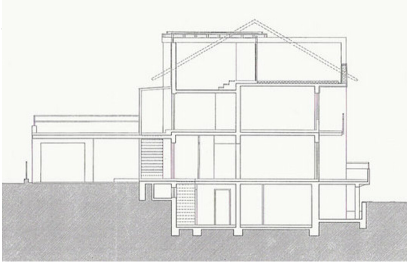
Haus Wald, Umbau
