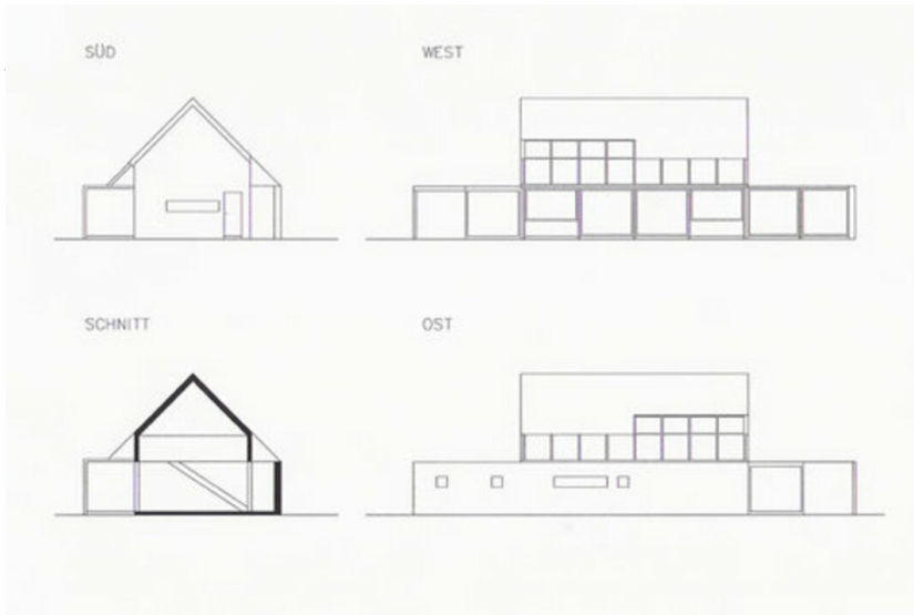
Ansichten, Schnitt
