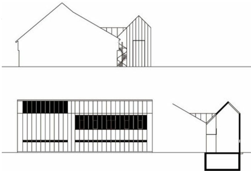
Ansichten, Schnitt
