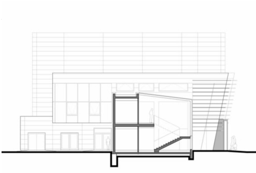
Schnitt Süd/Ost
