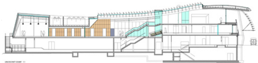
Schnitt
