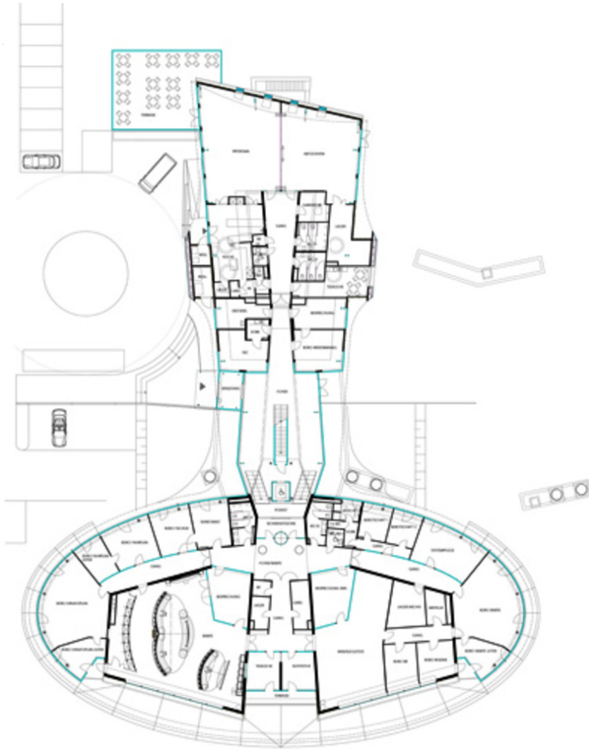
Grundriss
