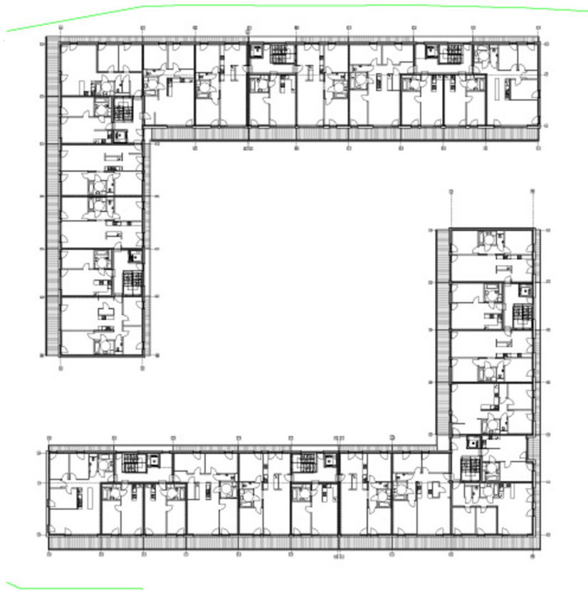
Grundriss RG
