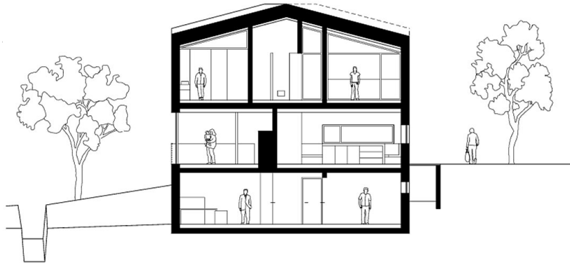
Querschnitt
