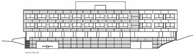
Ansicht Süd-Ost
