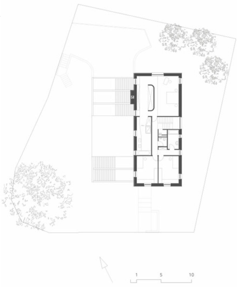
Grundriss OG
