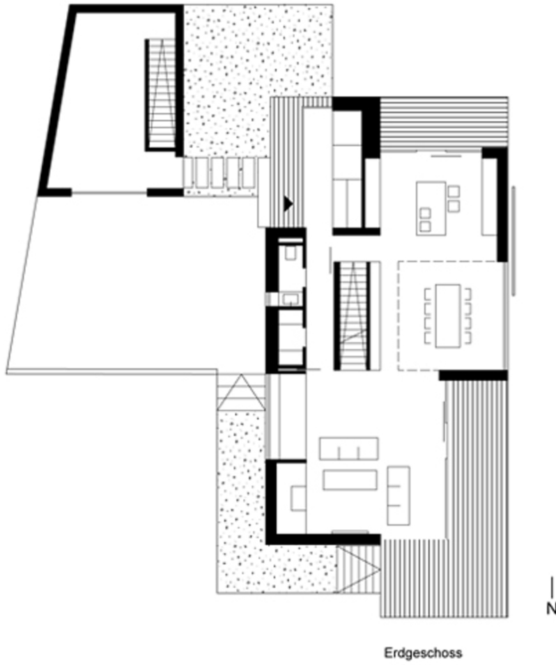
Grundriss EG
