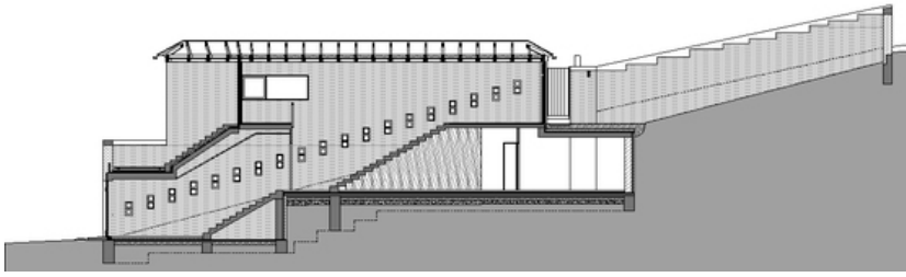
longitudinal section
