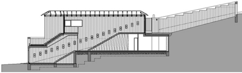
longitudinal section
