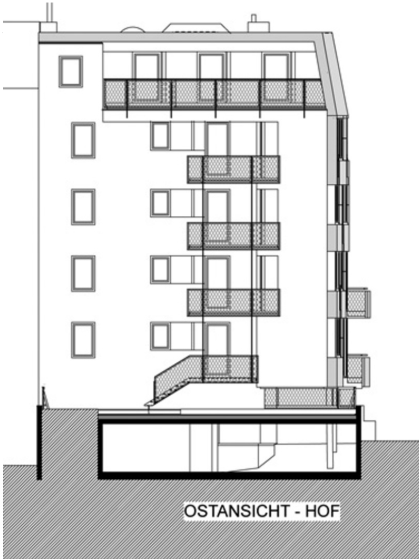
Ansicht Ost
